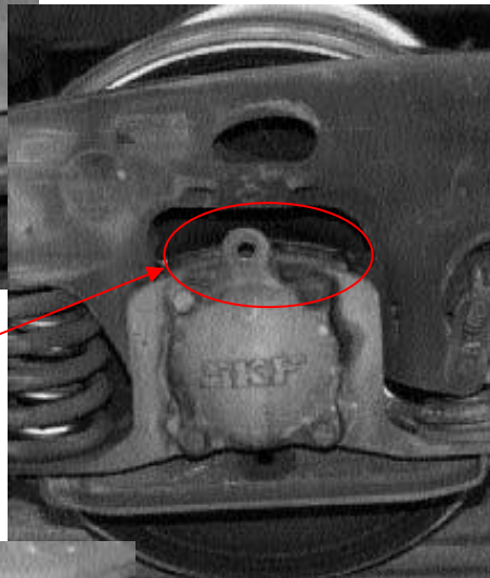
Fig. 7 Plaques d'usure manganèse bogies et de boites dessoudées
