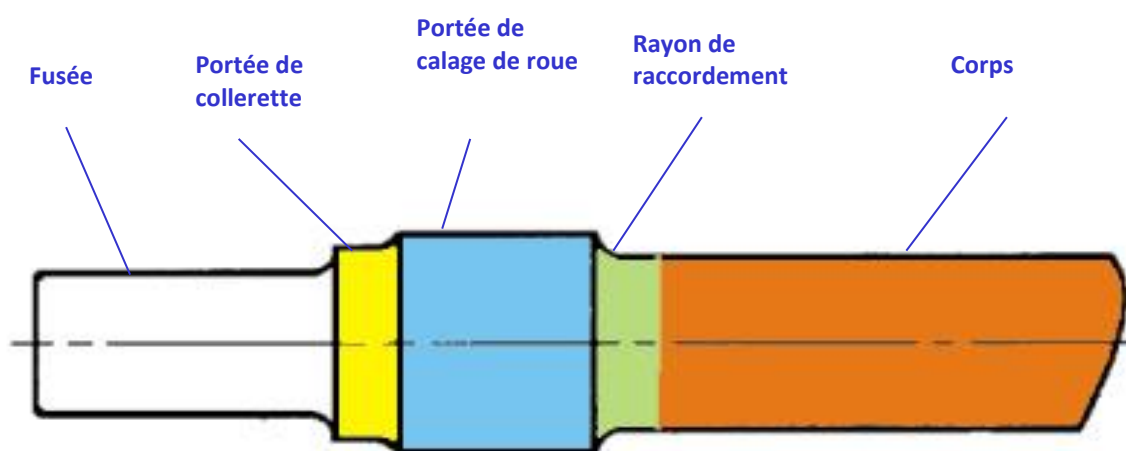
Exemple d'essieu-axe
